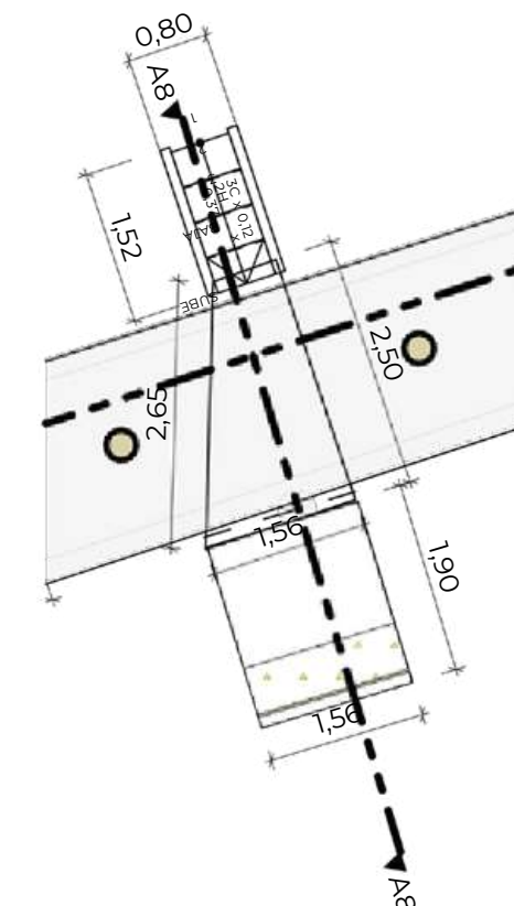
PLANTA DEL JUEGO 1 - ESCALAR Esc. 1:100
