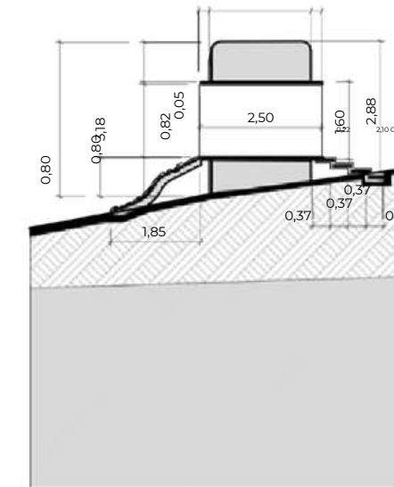
CORTE JUEGO 1 ESCALAR 1:100
