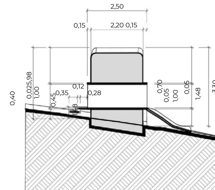
CORTE JUEGO 4 DEL RESBALIN Esc. 1:100
